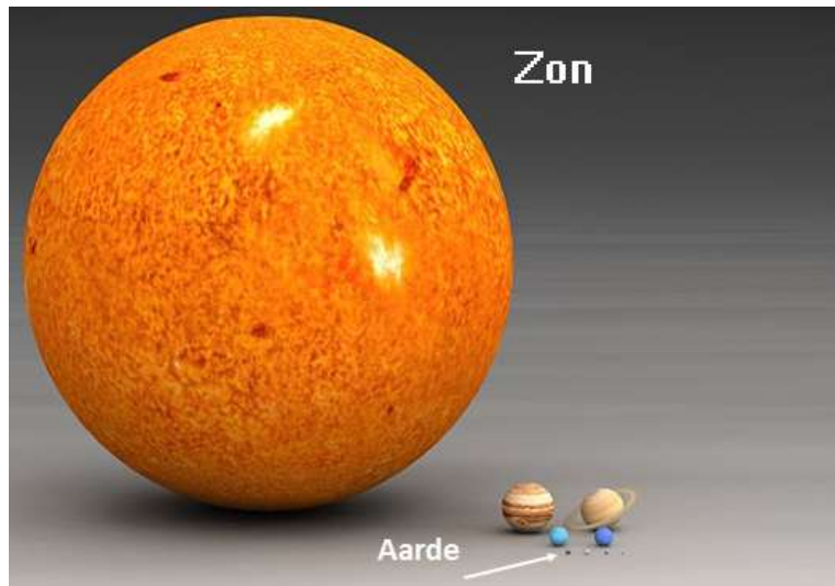
Fig. 1. De Zon in vergelijking met de planeten qua omvang. © CC-BY-SA 3.0 Ismpascal
