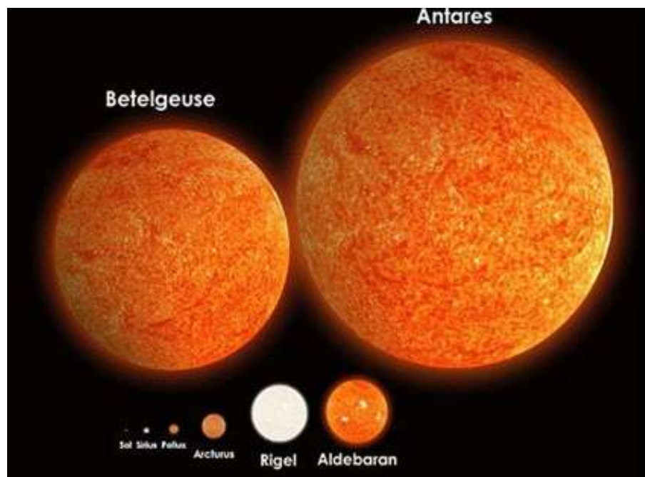
De echte reuzen op een rijtje: Aldebaran, Rigel, Betelgeuze en Antares. © CC-BY-SA 4.0, site: http://www.abovetopsecret.com/
