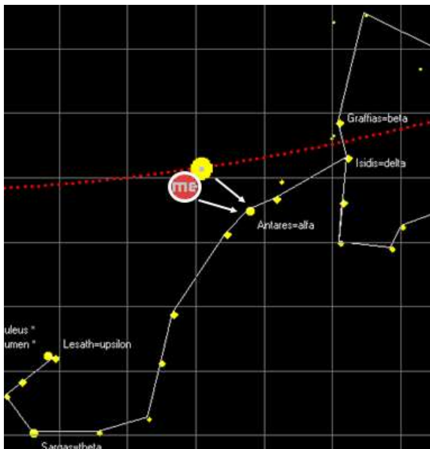
Zon en Mercurius samen conjunct de ster Antares - koning Charles-I
