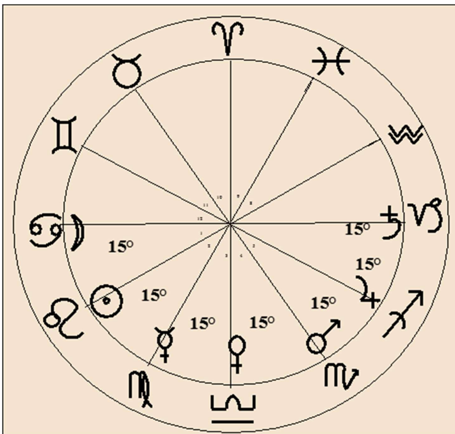
Fig.44. Het Thema Mundi, de geboorte van het universum.
