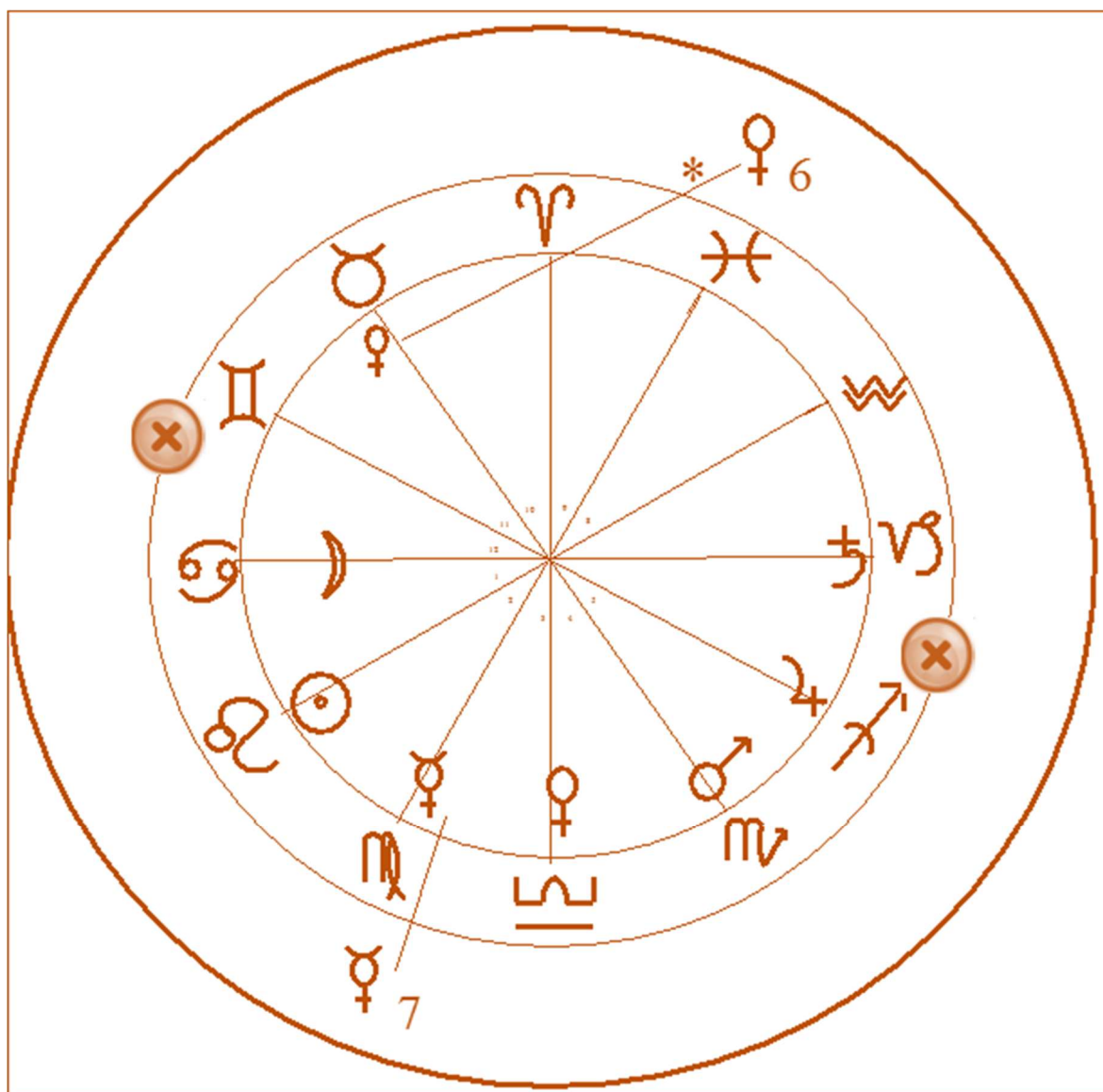
Fig. 47. De exaltaties van de planeten Venus en Mercurius.
