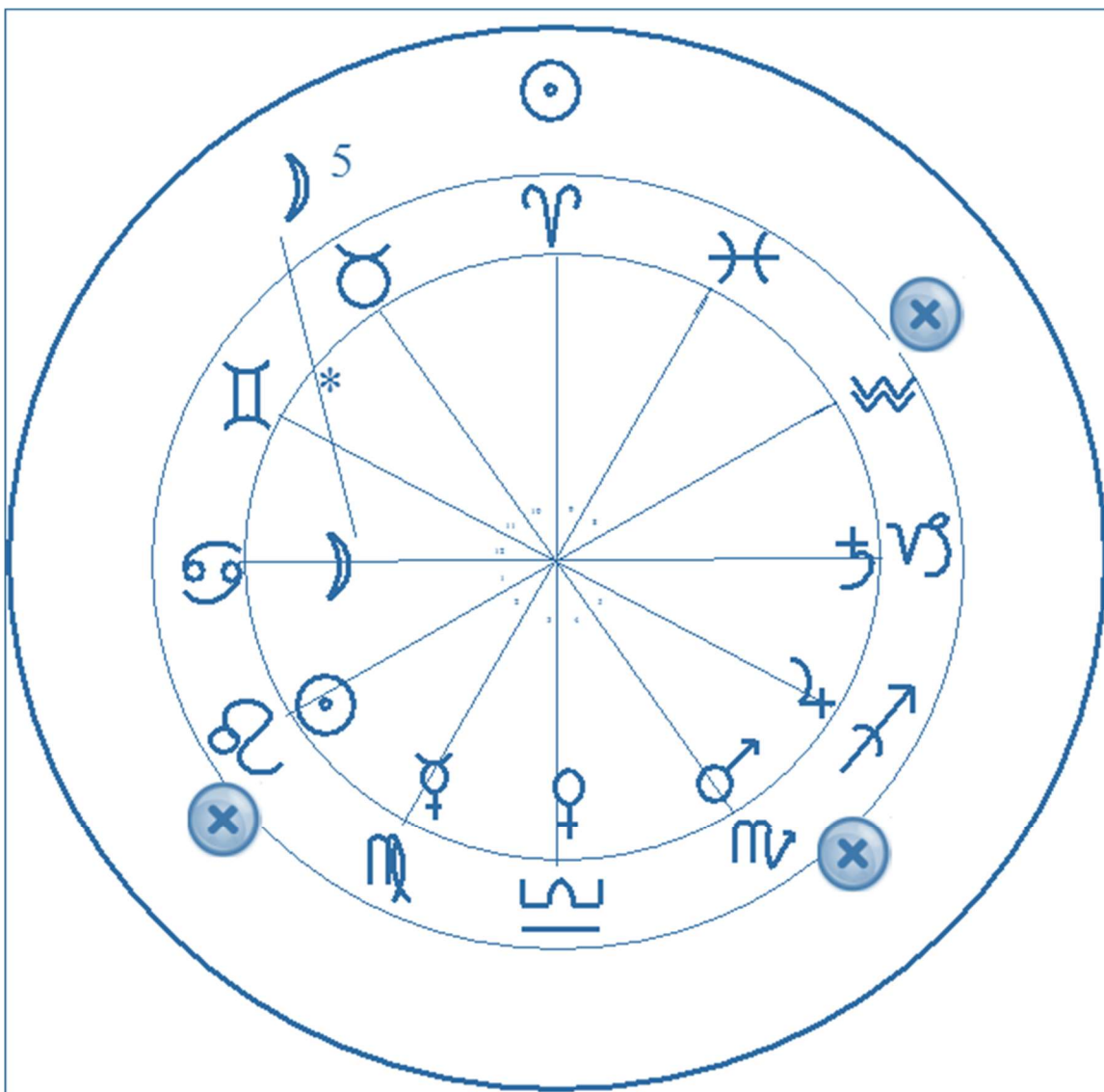
Fig. 46. De exaltatie van de Maan in het teken Stier.
