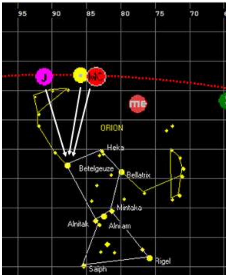
De vaste ster Betelgeuze in conjunctie met de Zon bij Paul Mc. Cartney.
