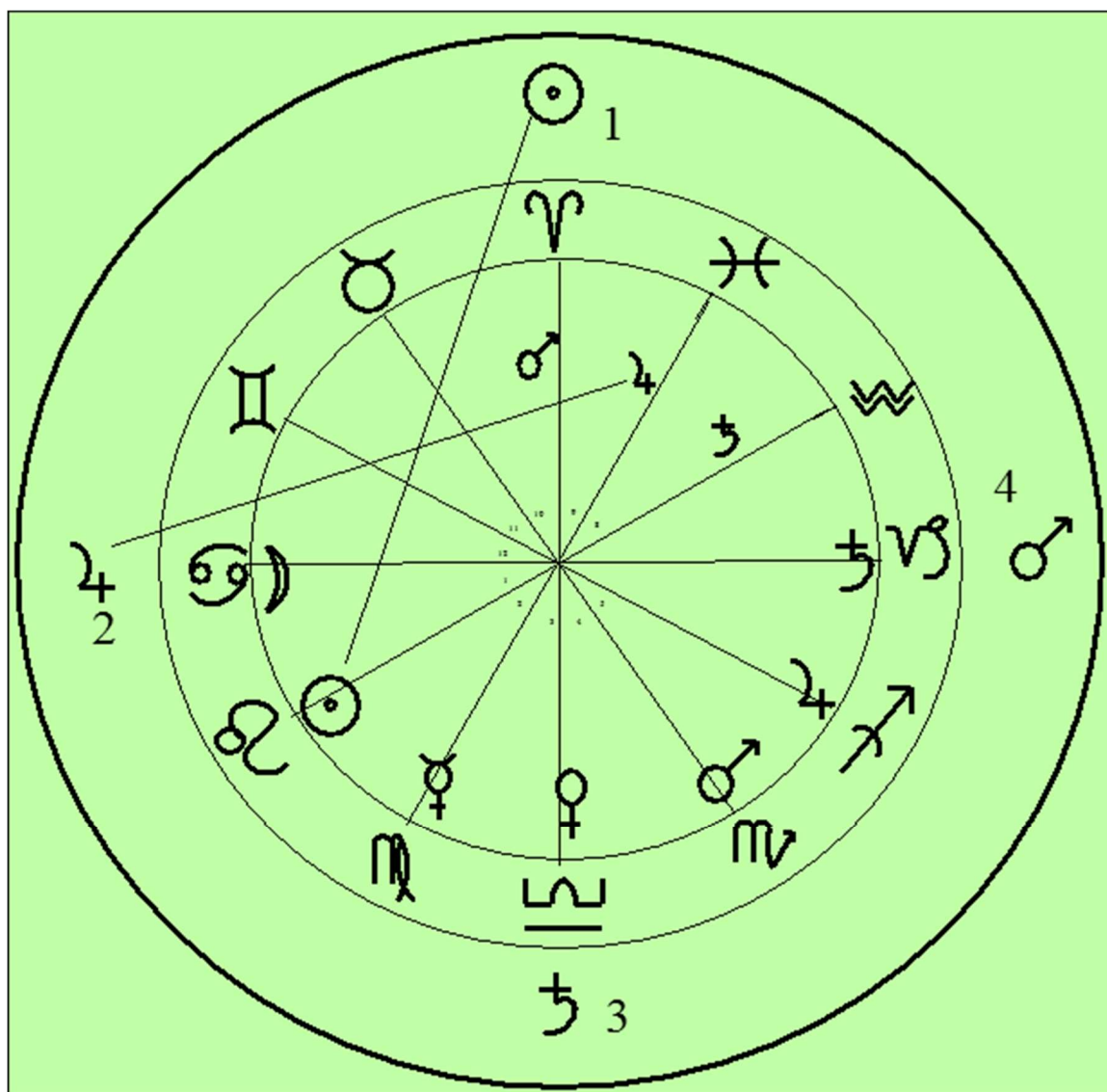
Fig.45. Thema Mundi en de exaltaties van de vier grootste planeten.
